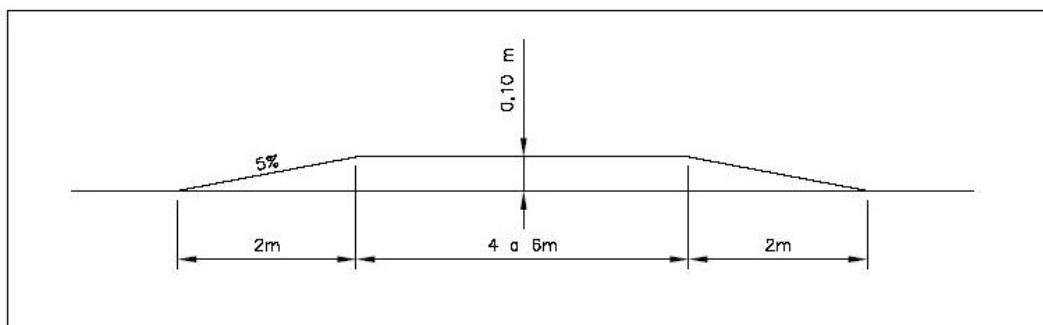
Pas de vianants de ressalt – Circular 02/05 de 14 de març de 2005
